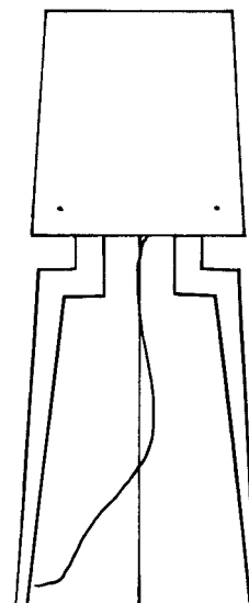
Zpindel bordlampa 622-1614 Ø skärm 160 h skärm 170 Reflektor vit plåt H 440 Sladd 2000 transp. E27 lamphållare Lågenergilampa (ingår)
