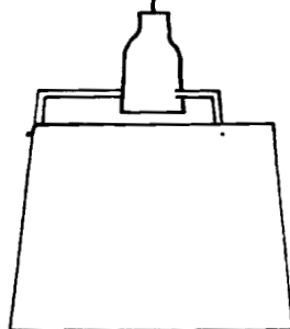
Zpindel pendel 656-2219 Ø skärm 220 h skärm 155 H 240
